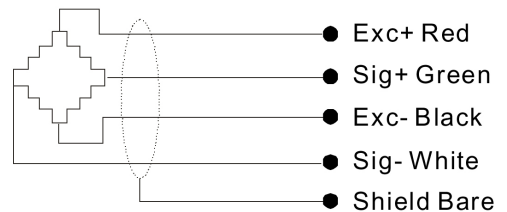
結線図
