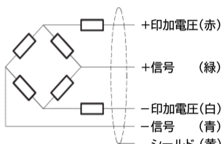
ケーブル接続図
