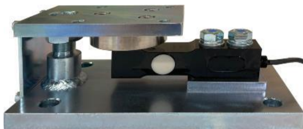
浮き上がり防止 (LU-OC)
