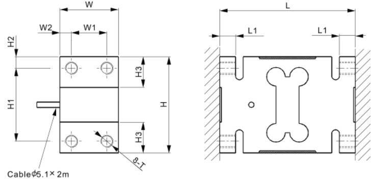
寸法図
